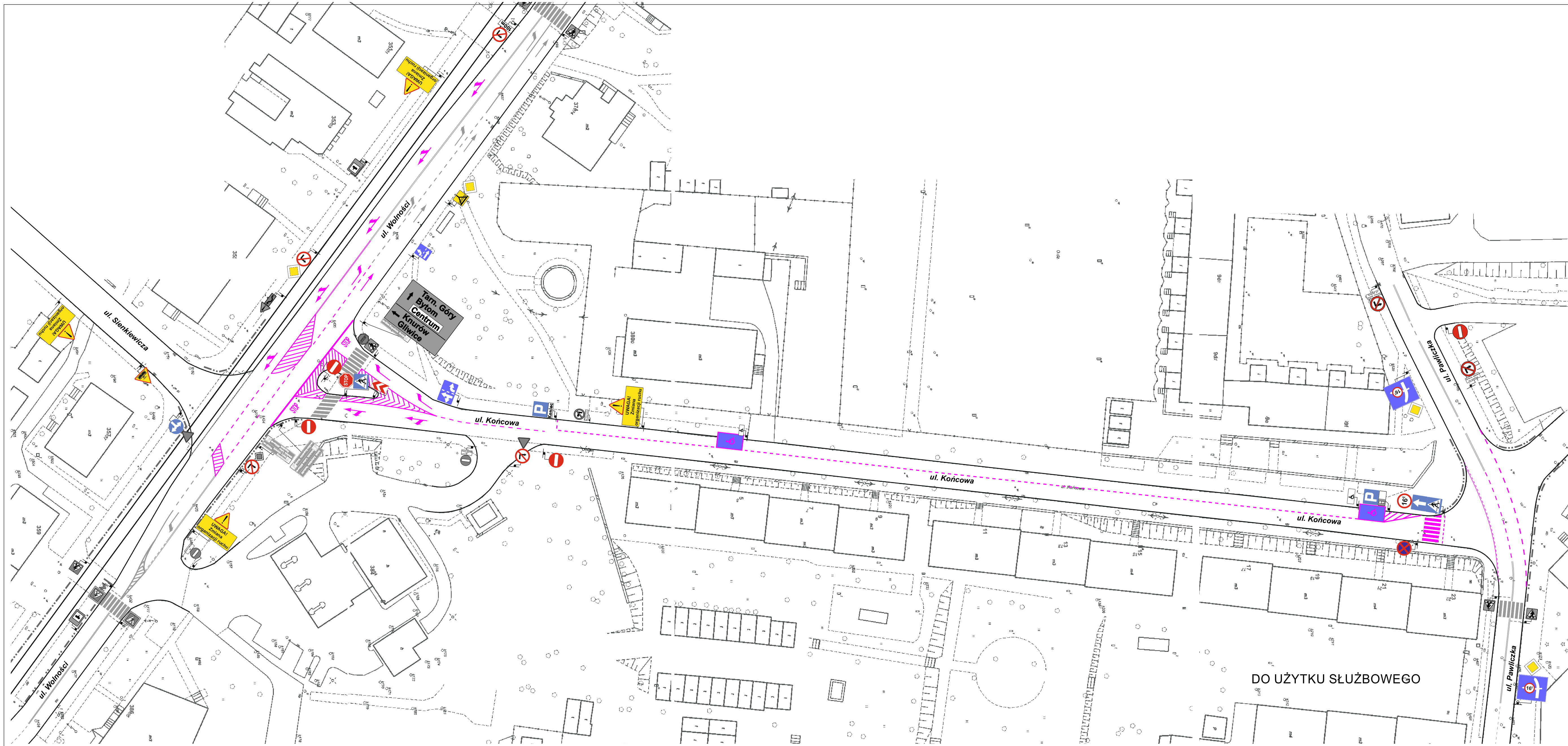
Projekt docelowej organizacji ruchu na ul. Końcowej - wprowadzenie jednego kierunku ruchu oraz ograniczeń tonażowych. skala 1:500
